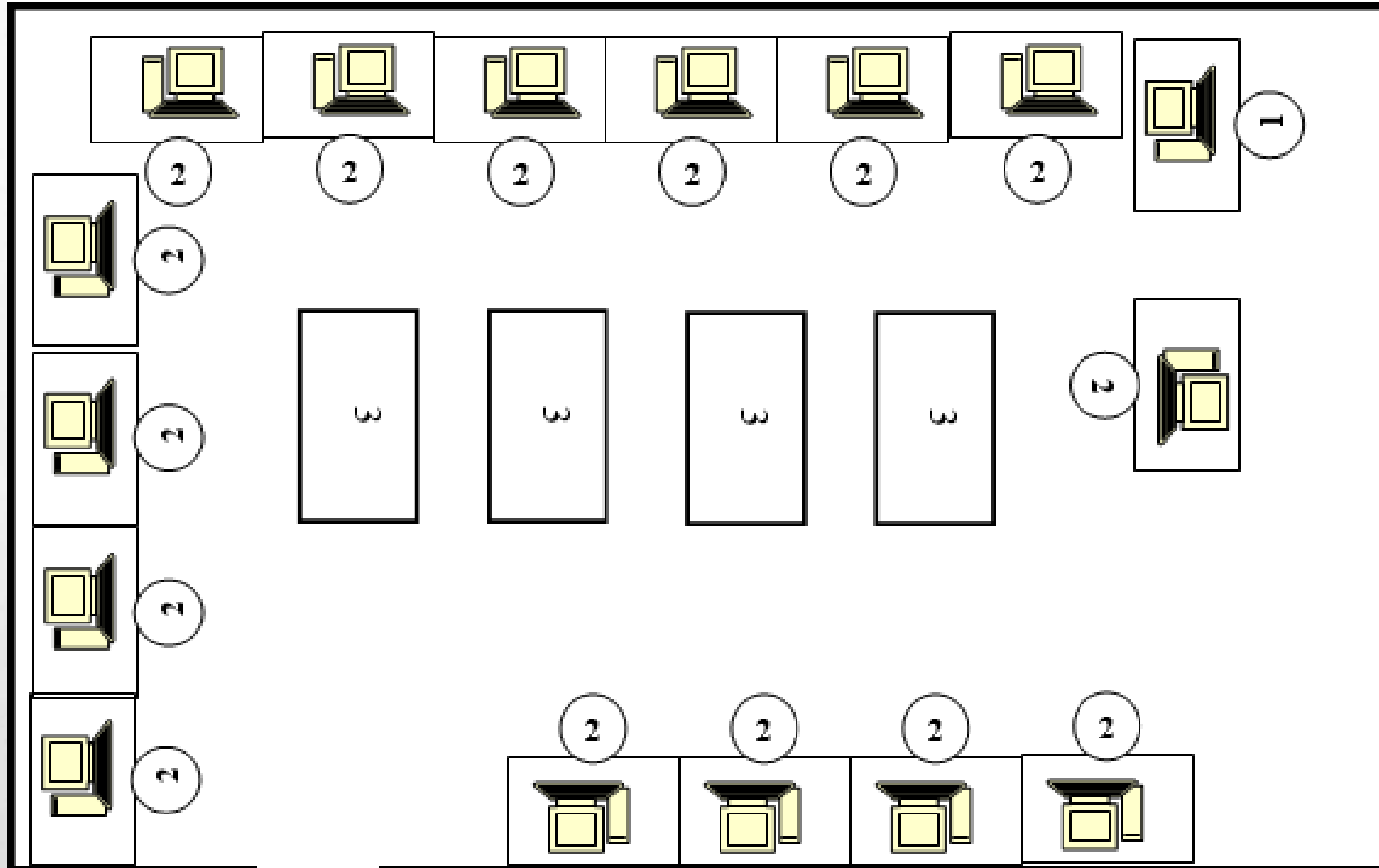
рис. 5.5 Схема кабінету інформатики, де: 1 – комп'ютерний стіл учителя; 2 – комп'ютерний стіл учня; 3 – парти.
